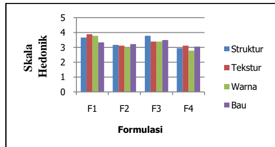
Gambar 2. Mutu Organoleptik Struktur, Tekstur, Warna dan Bau Remah Rotidari Formulasi Mocaf 0% (F1), 10% (F2), 20% (F3) dan 30% (F4). Skala 1=sangat tidak suka; 2=tidak suka; 3=agak suka;4=suka; 5=sangat suka
